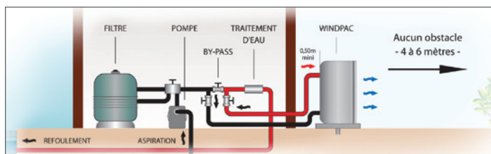
Schéma d'installation
